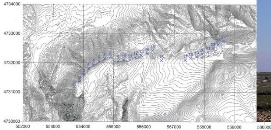
Figura 4. Posiciones de setogenerador para el proyecto P.E. Cruz de Aldea.
